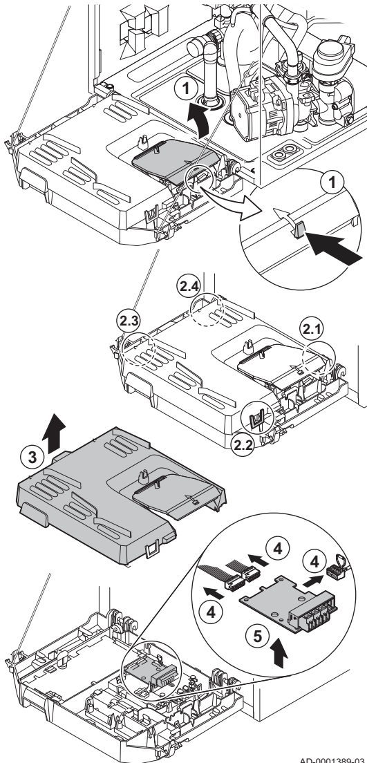
Abb.110 Zugang zu den Anschlüssen
