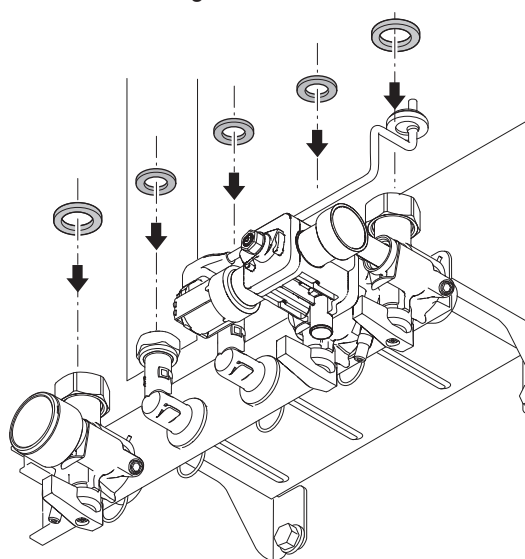
Abb.12 Dichtungen montieren
