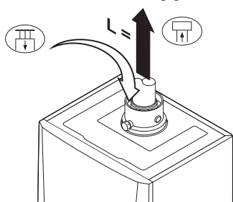
Abb.21 Raumlufthängige Version
