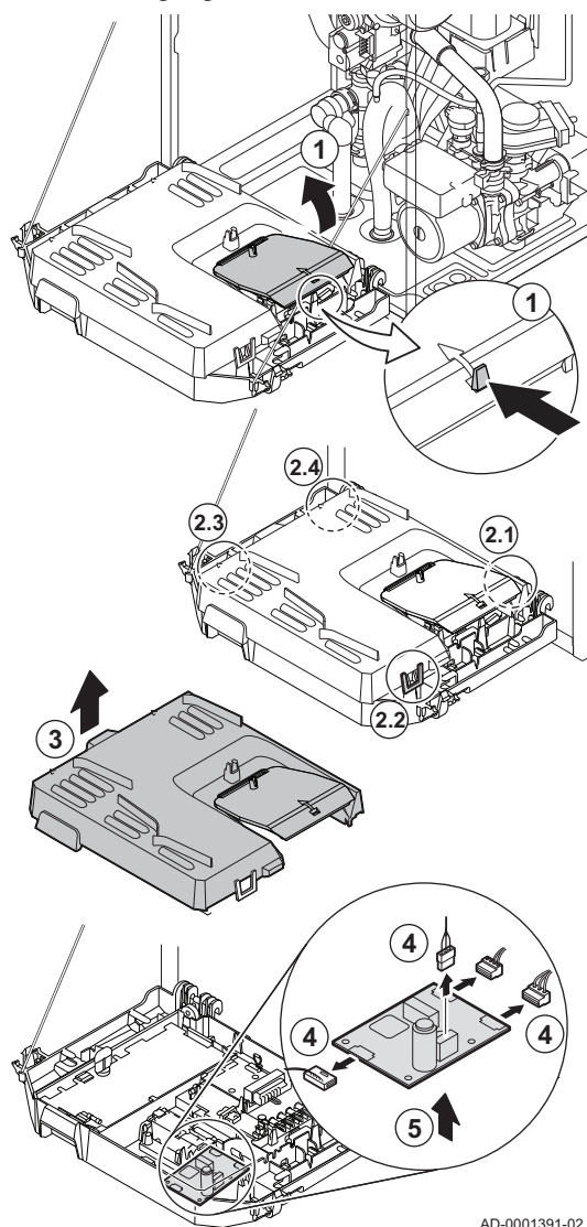
Abb.111 Zugang zu den Anschlüssen
