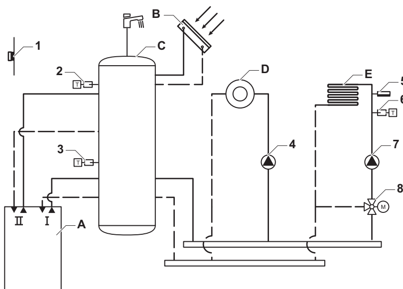
Abb.56 1 Kessel + 1 Kombi-Pufferspeicher + 1 ungemischter Kreis + 1 Mischerkreis + Sonnenkollektoren
