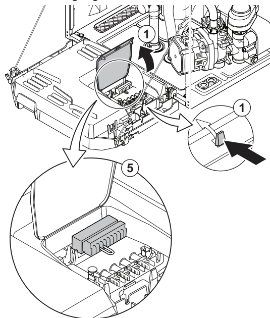
Abb.28 Zugang zu den Anschlüssen
