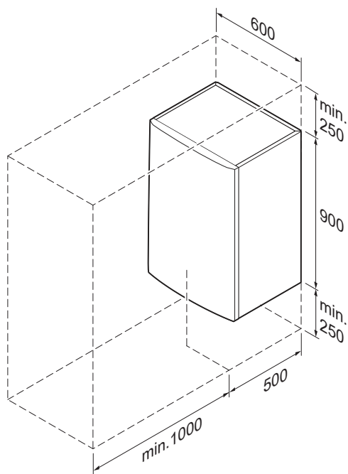
Abb.8 Installationsbereich
