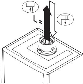
Abb.24 Raumluftunabhängige Ausführung
