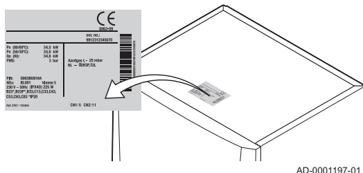
Abb.7 Lage des Typenschilds
