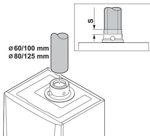
Abb.27 Anschluss des Abgasstutzens und der Luftzufuhr
