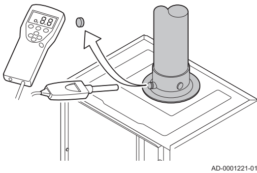
Abb.66 Abgasmesspunkt
