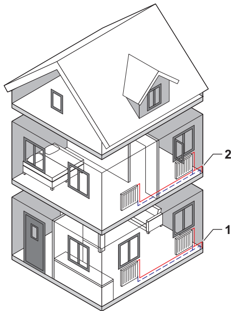
Abb.78 Zwei Heizkreise
