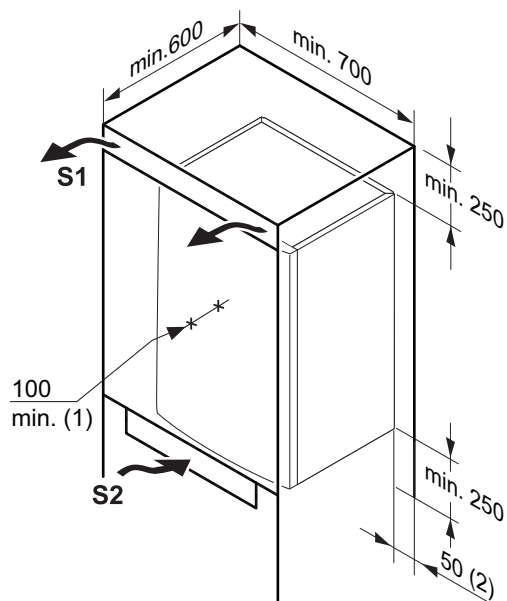
Abb.9 Platz für Belüftung
