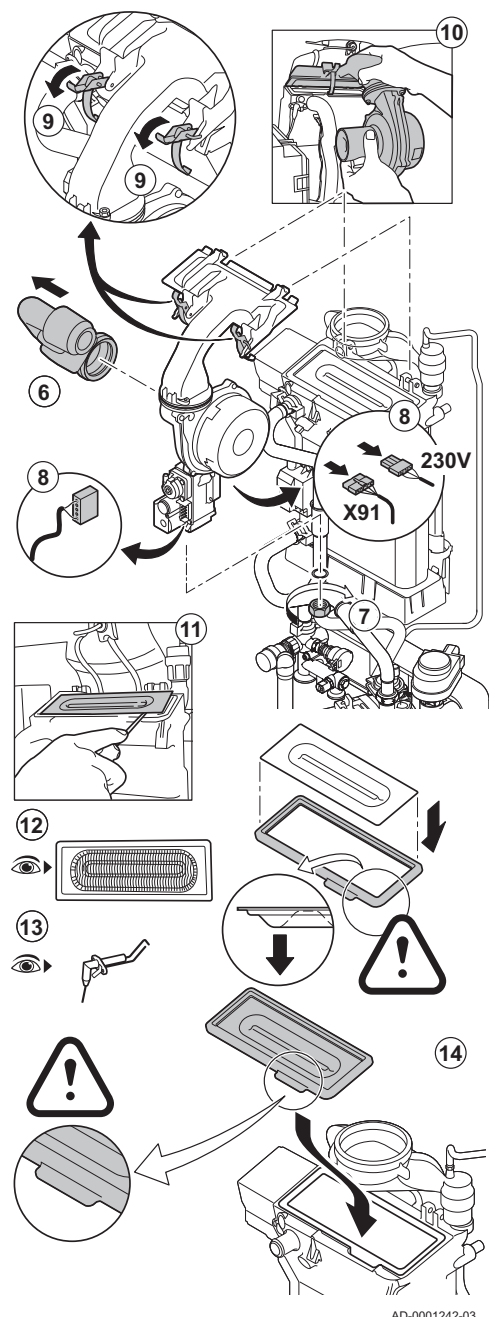
Abb.101 Überprüfung des Brenners
