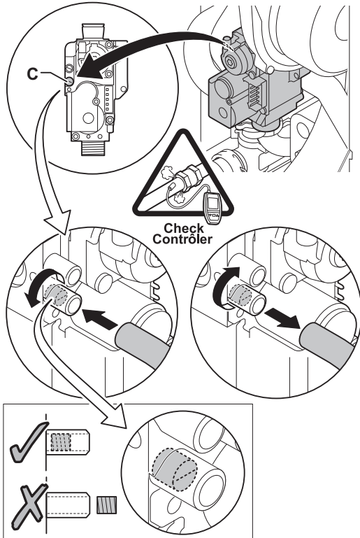
Abb.64 Prüfoffnungen der Gasventilbaugruppe
