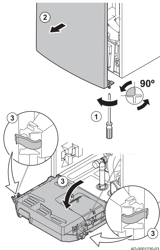
Abb.102 Öffnen des Heizkessels
