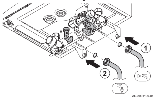
Abb. 15 Trinkwasserseitige Anschlüsse
