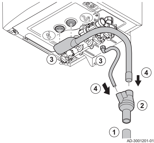
Abb.16 Anschluss der Kondensatleitung
