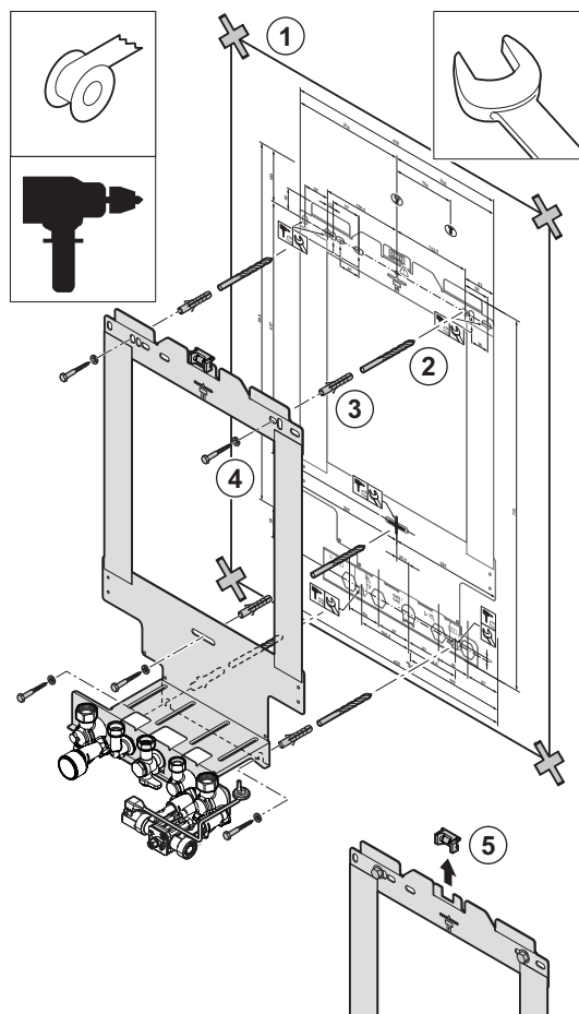
Abb.10 Anbringung des Montagerahmens
