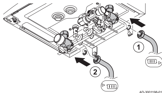
Abb. 14 Anschluss des Heizkreises
