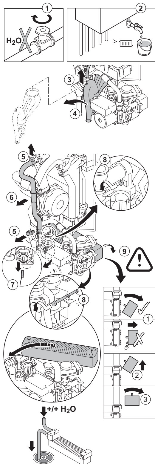
Abb.104 Reinigen des Plattenwärmetauschers
