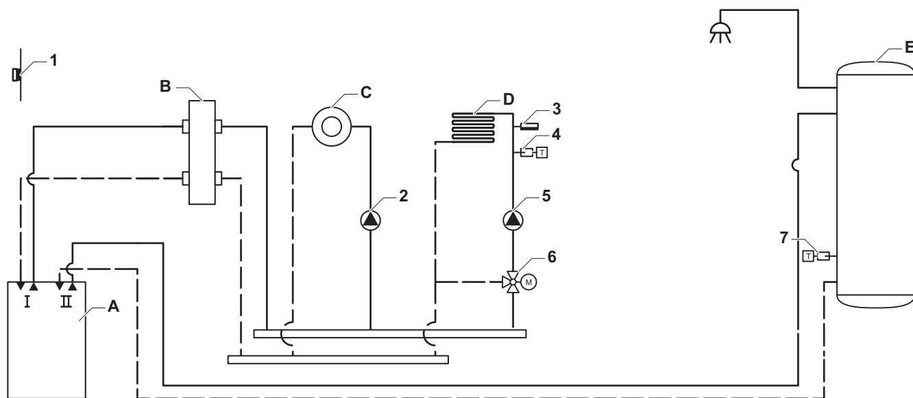
Abb.52 1 Heizkessel + 1 LLH + 1 ungemischter Kreis + Mischerkreis + TWW-Kreis
