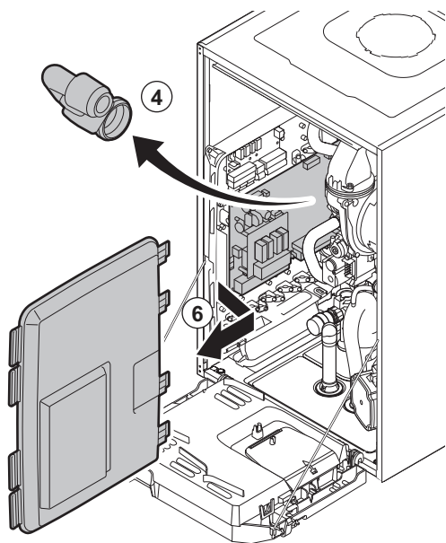
Abb.37 Zugang zur Leiterplatte
