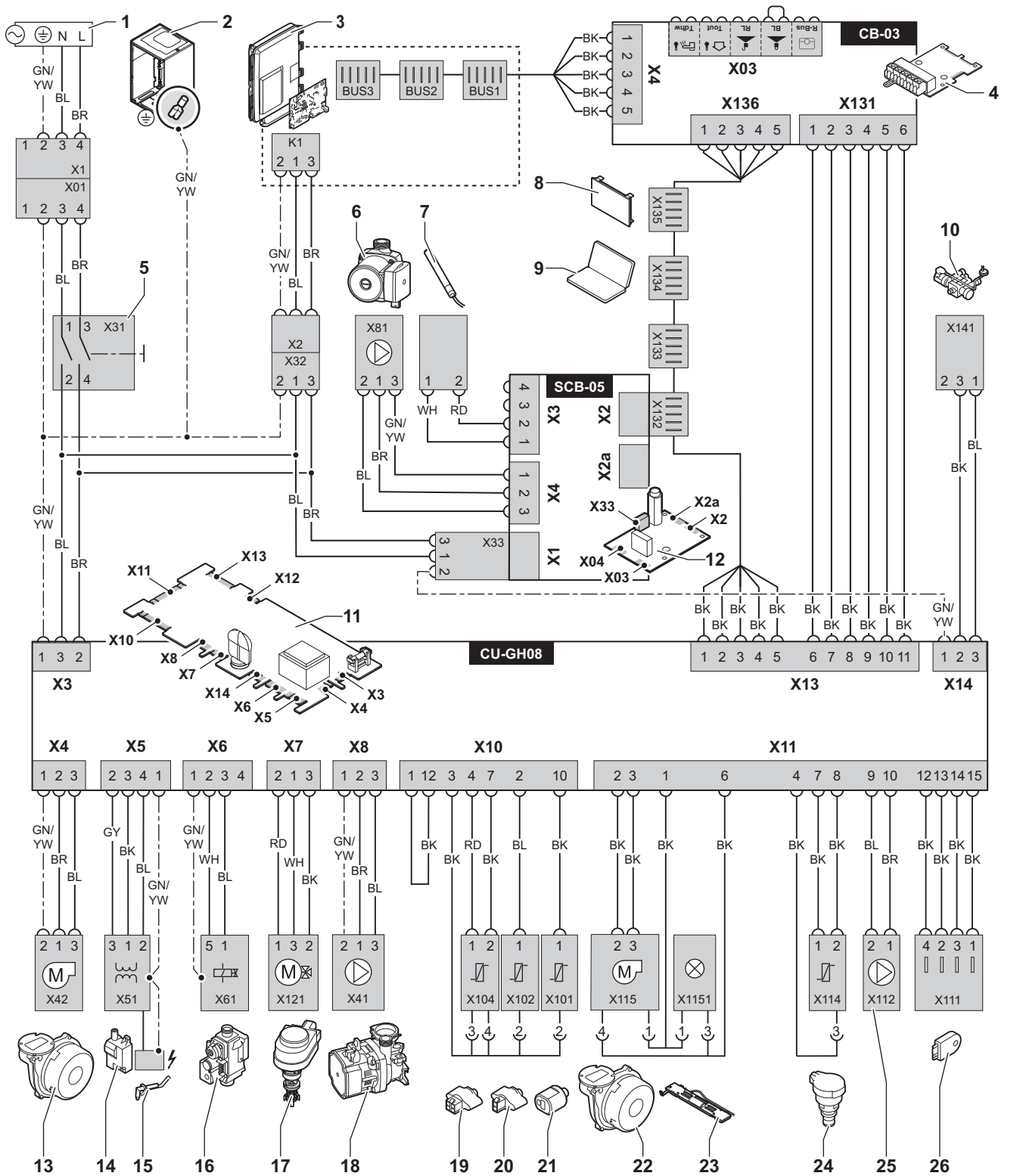
Abb.2 Elektrischer Schaltplan
