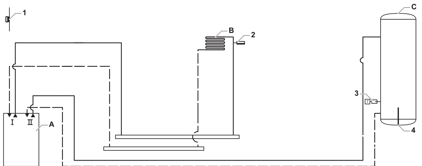
Abb.50 1 Heizkessel + 1 ungemischter Kreis + WW-Kreis
