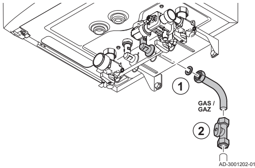
Abb.17 Anschluss der Gasleitung
