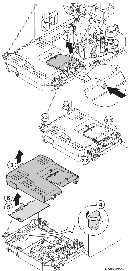
Abb.109 Zugang zu den Anschlüssen
