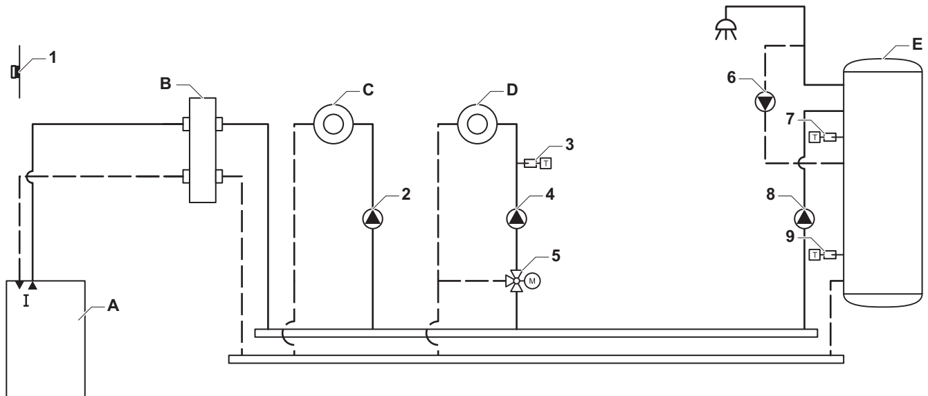
Abb.53 1 Kessel + 1 hydraulische Weiche + 1 ungemischter Kreis + Mischerkreis + TWW-Kreis
