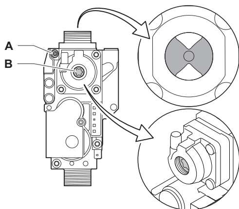
Abb.72 Einstellschraube A
