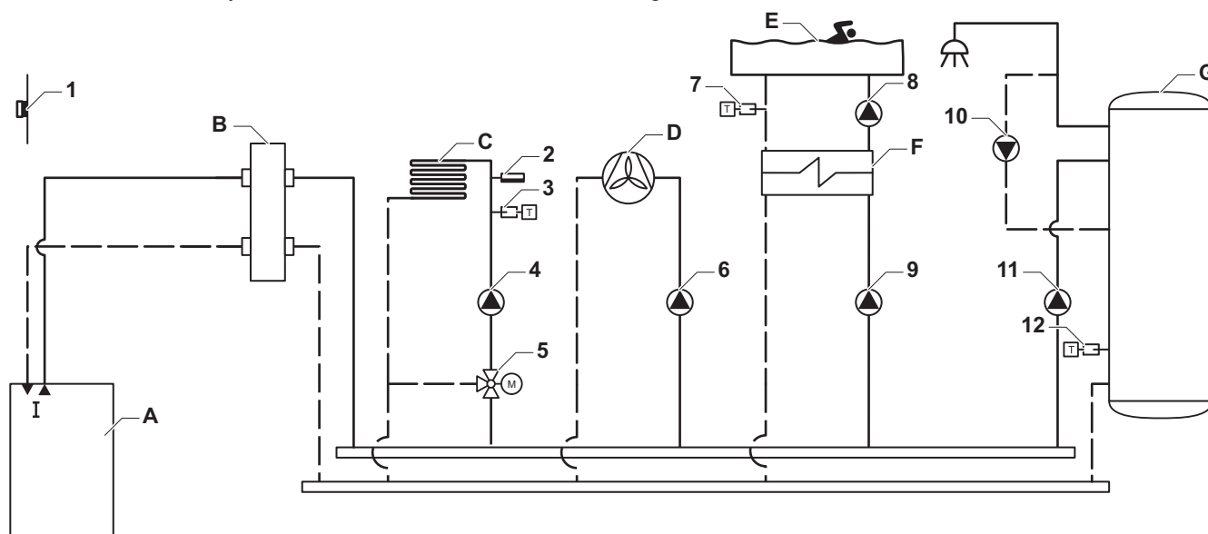
Abb.54 1 Kessel + 1 hydraulische Weiche + 1 Mischerkreis + 1 ungemischter Kreis + Schwimmbad + TWW-Kreis
