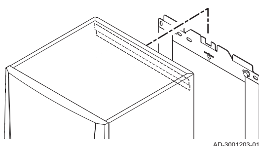
Abb.13 Kessel montieren
