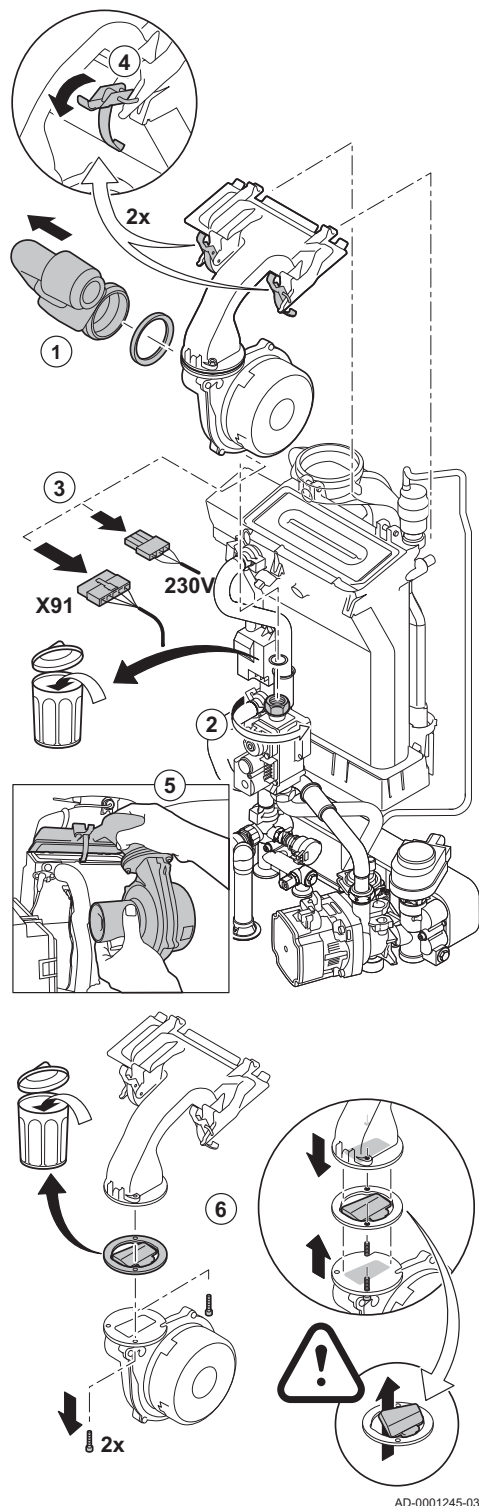
Abb.108 Auswechseln der Rückstromsicherung
