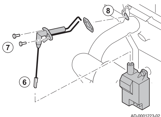
Abb.103 Austausch der Ionisations- und Zündelektrode
