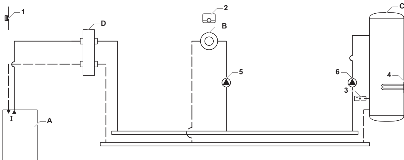
Abb.51 1 Kessel + 1 hydraulische Weiche + 1 ungemischter Kreis + TWW-Kreis mit elektrischem Heizelement
