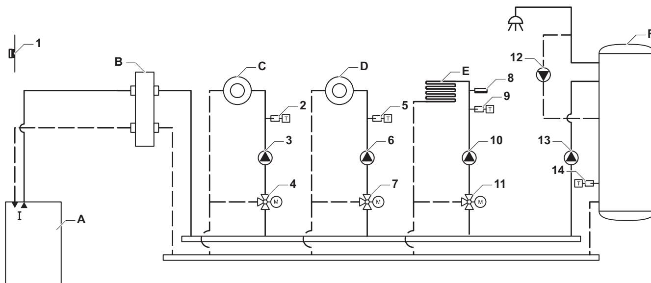
Abb.55 1 Kessel + 1 hydraulische Weiche + 3 Mischerkreise + TWW-Kreis
